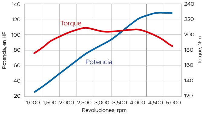
CARACTERÍSTICA TORQUE-VEOLCIDAD
